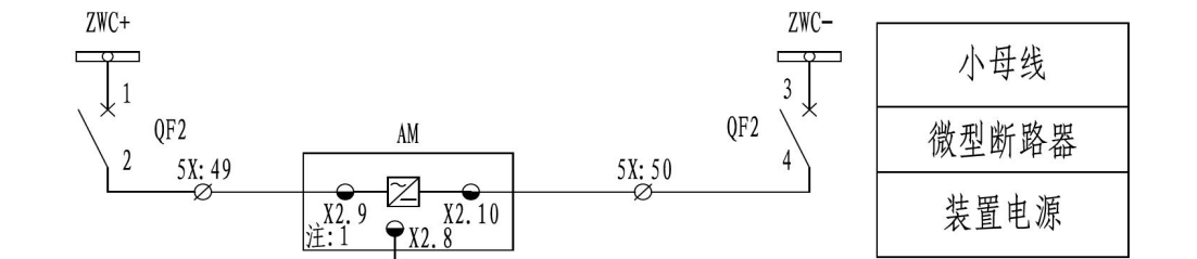
图 1.20 AM3SE-I 二次原理图（一）
