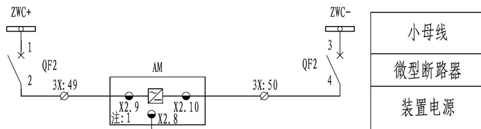
图 2.7 AM3SE-U 二次原理图 (一)
