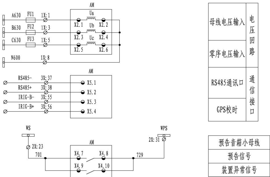
图 2.9 AM3SE-U 二次原理图（三）
