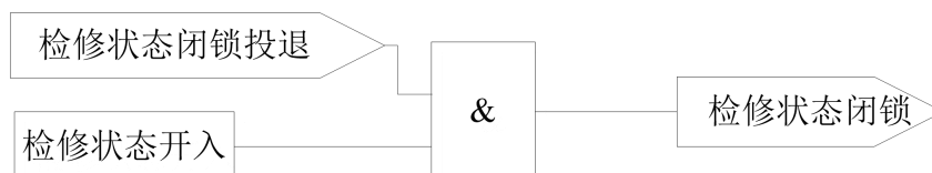
图 1.17 检修状态闭锁逻辑
