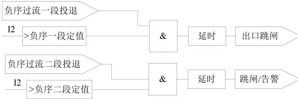
图 1.12 两段式负序过流保护逻辑
